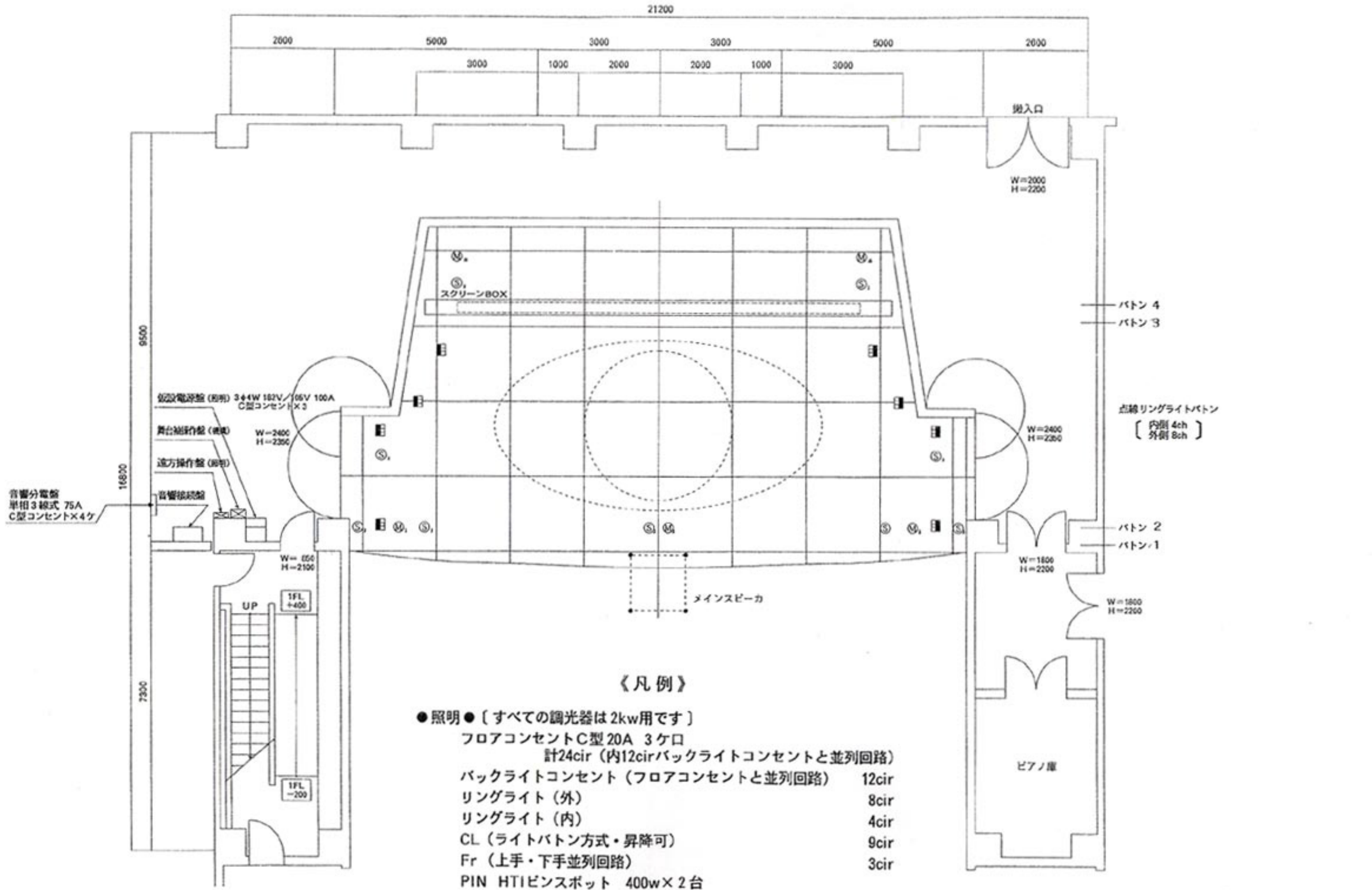
レザンホール (塩尻市文化会館) 中ホール舞台平面図 縮尺 1:100 方眼目盛=1.818m (1間)
